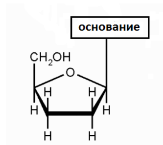
Дидезоксинуклеозид
