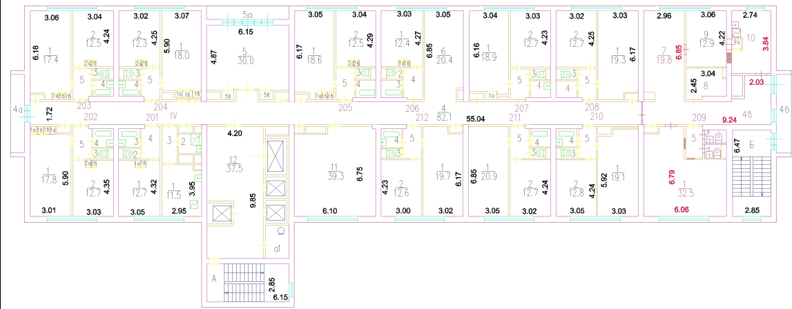
2 этаж Головинское шоссе., д.8, корп.1
