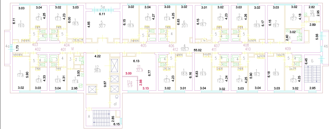
4 этаж Головинское шоссе., д.8, корп.1
