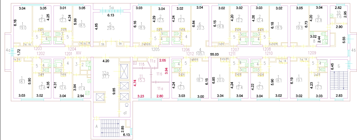
12 этаж Головинское шоссе., д.8, корп.1
