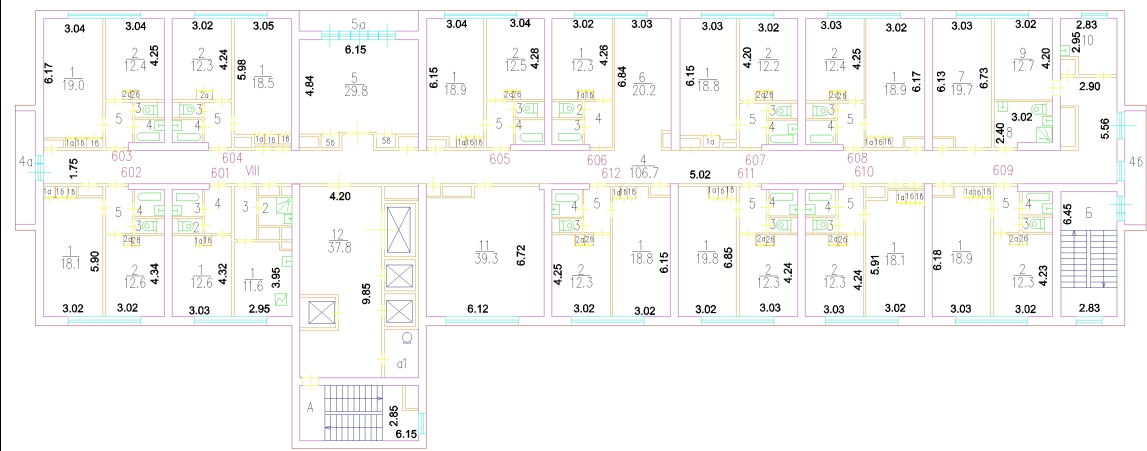
6 этаж Головинское шоссе., д.8, корп.1
