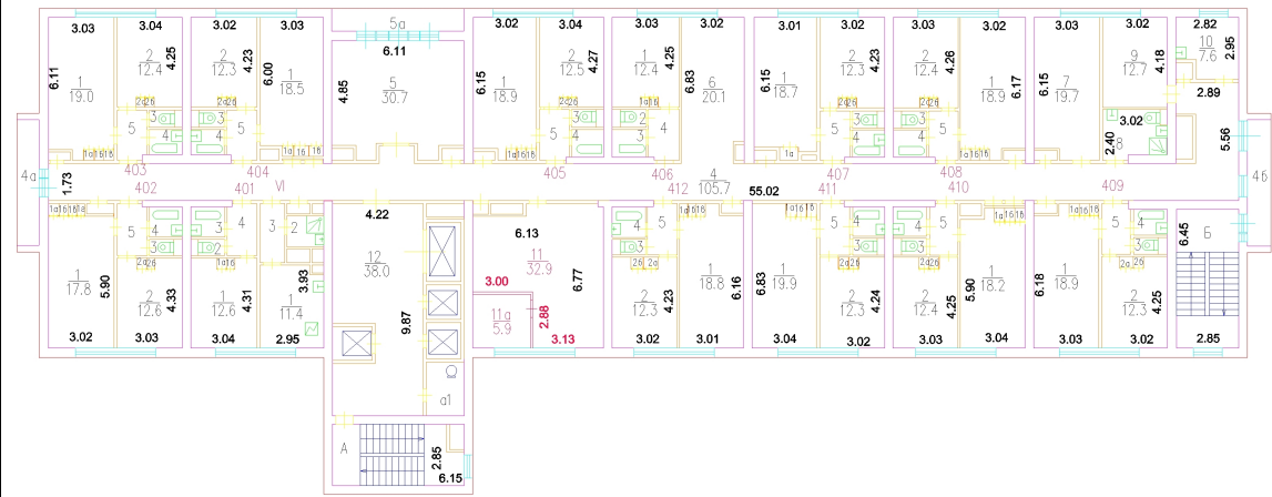
4 этаж Головинское шоссе., д.8, корп.1
