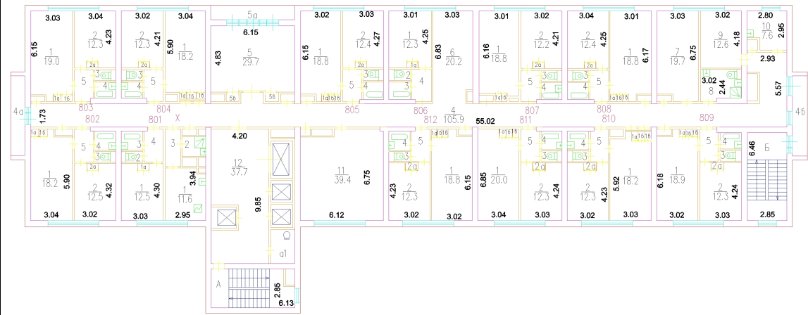
8 этаж Головинское шоссе., д.8, корп.1
