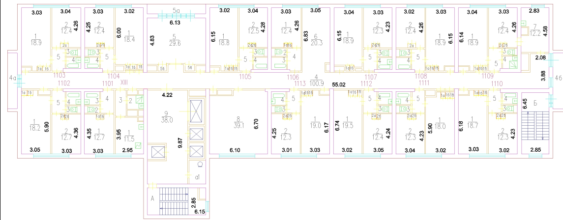
11 этаж Головинское шоссе., д.8, корп.1
